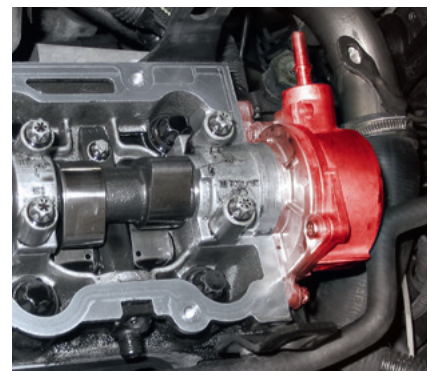
Vakuumpumpe und Nockenwelle im Opel Vectra B (hervorgehoben)
