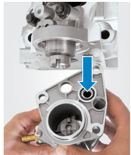
Ölversorgung über den Flansch z. B. Peugeot, Citroën mit 1.8/1.9 l Dieselmotor
